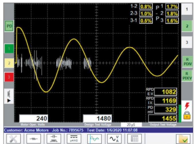
Регистрация частичного разряда
